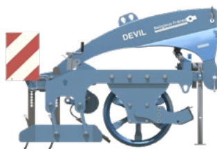
ROULOSANGE Ø600 Rouleau trapèze de 600 mm (carré de 40mm sur diagonale) + dents CROSS-BOARD et dents rigides.
