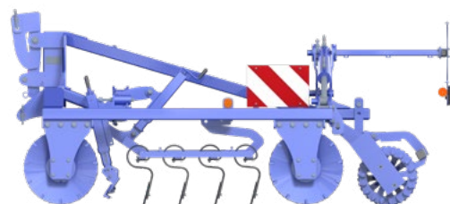
COMDOR P - MINI CROSKILL ROLPAF Ø410 + Kit éclairage.
