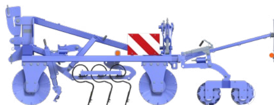
COMDOR P - ROTO-HERSE Ø300 + Équipement dents 32x12 + Kit éclairage
